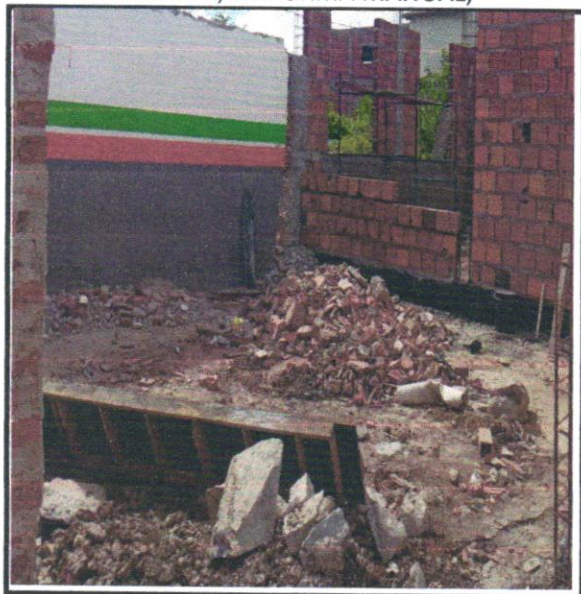
FOTO - 07 DEMOLIÇÃO DE PISO DE CONCRETO SIMPLES, DE FORMA MANUAL,
