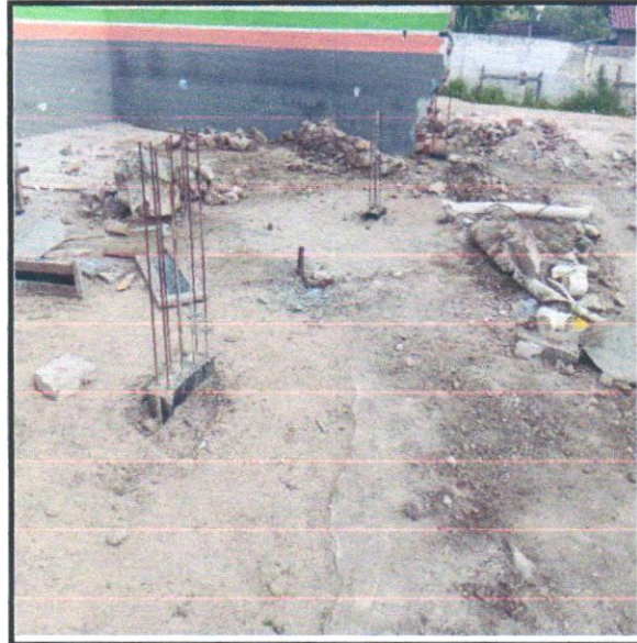
FOTO - 02 :DEMOLIÇÃO DE PISO DE CONCRETO SIMPLES, DE FORMA MANUAL, SEM REAPROVEITAMENTO. AF_09/2023
